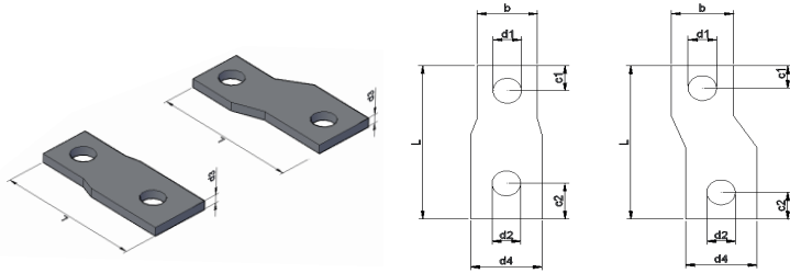
Kompakt Uzatma Barası (3mm)
