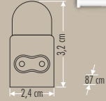
CT-2469 T5 BANT ARMATÜR BEYAZ KASA
