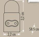
CT-2468 T5 BANT ARMATÜR BEYAZ KASA
