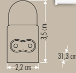
CT-2467 T5 BANT ARMATÜR BEYAZ KASA
